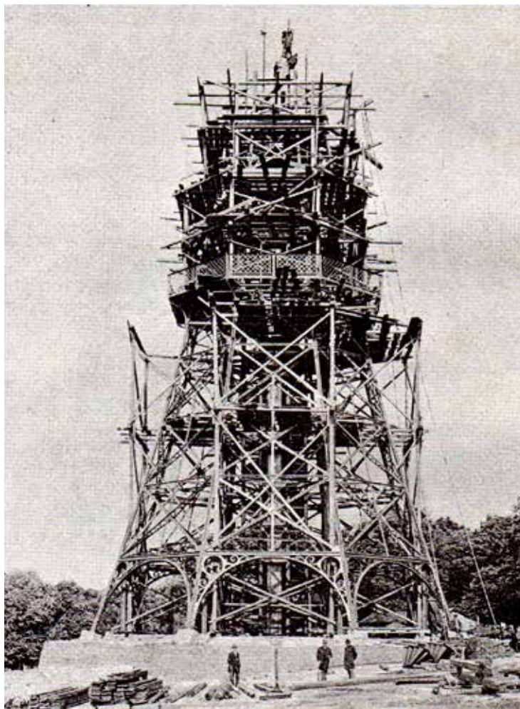
Rozestavěná Petřinská rozhledna, stav dne 13. června 1891 (foto: archiv KČT)
